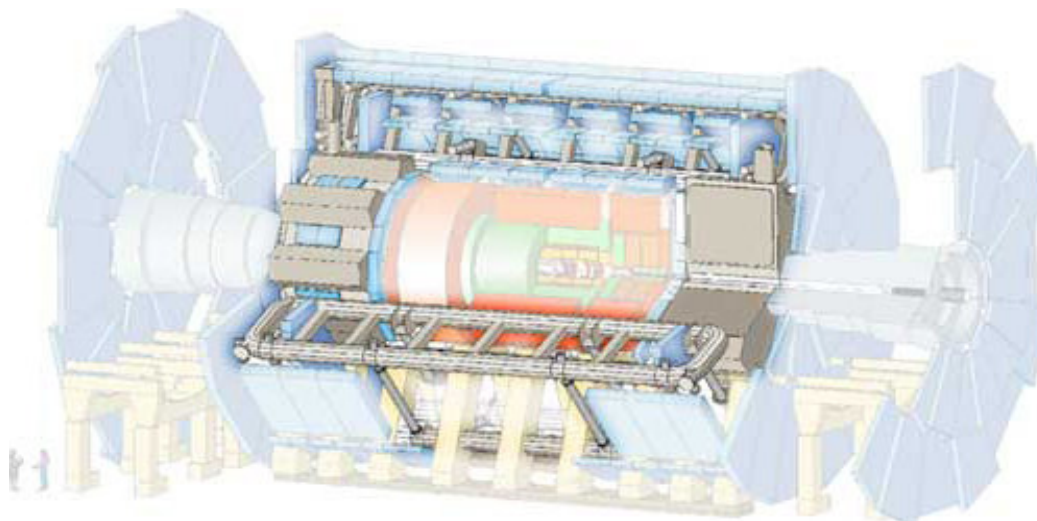
Σύστημα μαγνητών
